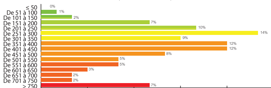
Figure 3 : Répartition 2018 des bâtiments de bureaux par consommation énergétique en énergie primaire selon l'échelle DPE (kWh EP /m 2 .an) (Source : OID 2018)
